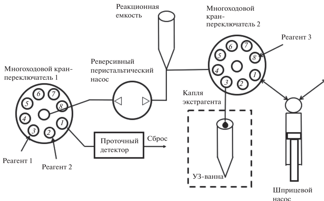
Рис. 5. Аэрогидравлическая схема циклического инъекционного анализа, включающая парофазную капельную микроэкстракцию.
